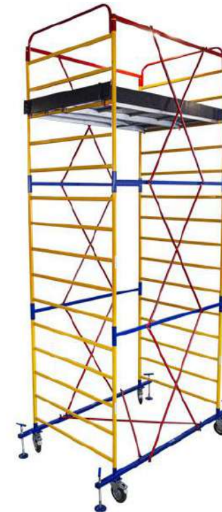
Вишка-тура «PROFITECH» з робочим майданчиком 2,0 x 1,35 м
